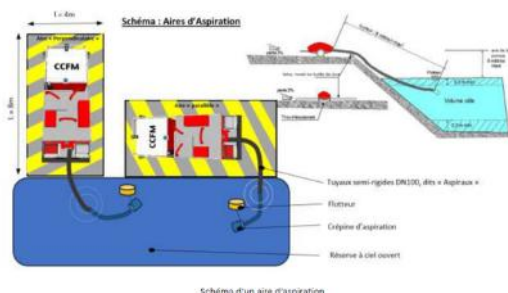
Schéma d'une aire d'aspiration
